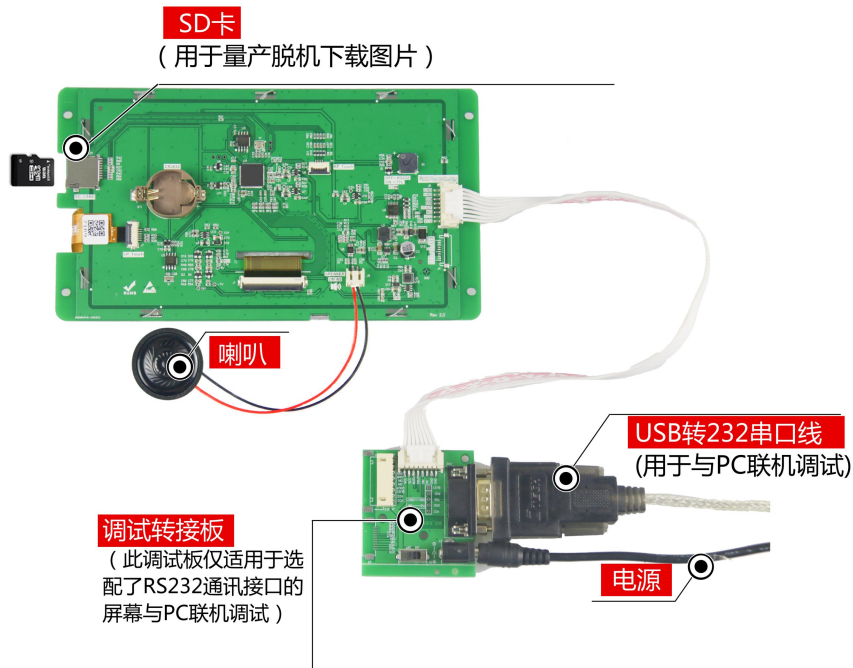
图 1-5 调试工具图
